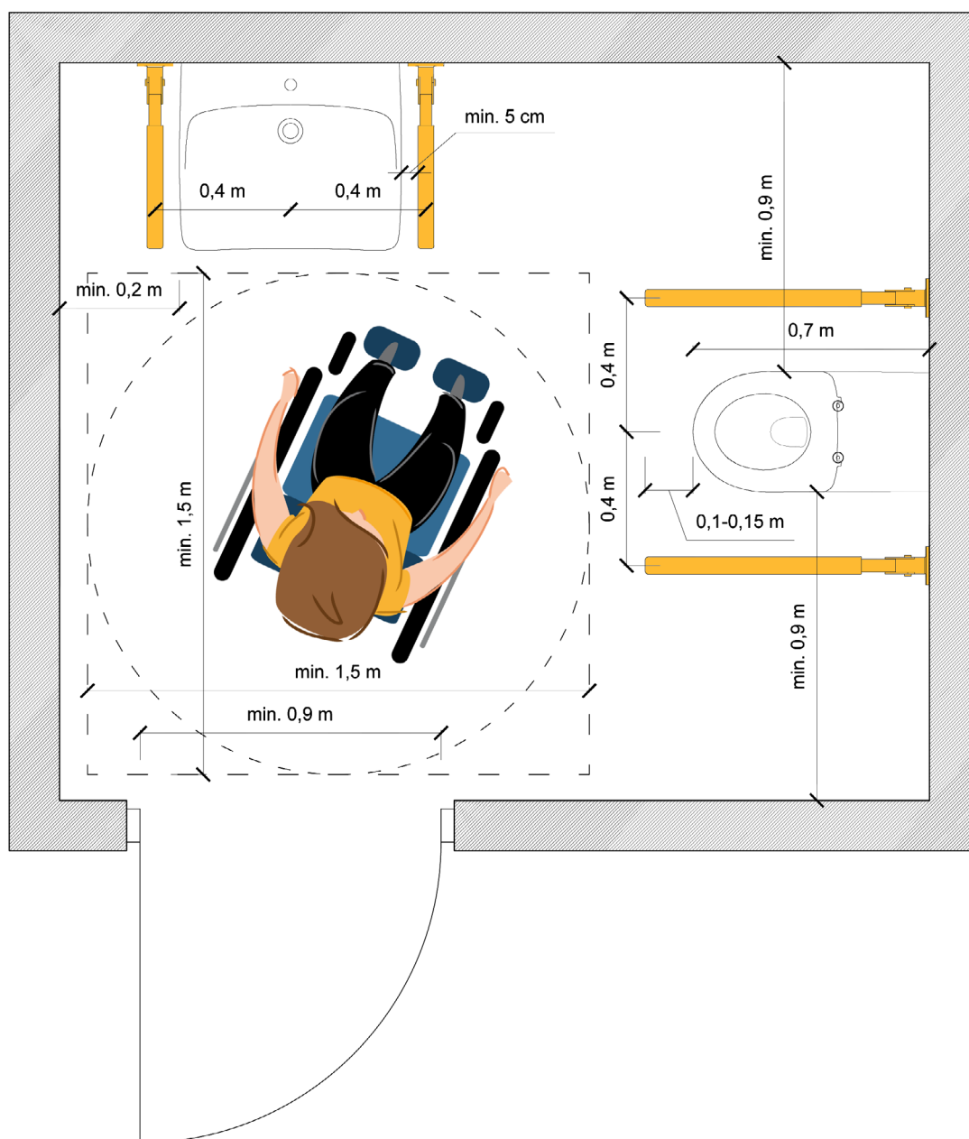
Ilustracja 77. Przykład rozmieszczenia sprzętów oraz powierzchni manewrowej i transferowej w toalecie przeznaczonej dla osób ze szczególnymi potrzebami, rys. Katarzyna Guratowska i Maria Görlich-Opyd (opracowanie własne na podstawie „Modelu Dostępnej Szkoły”)
