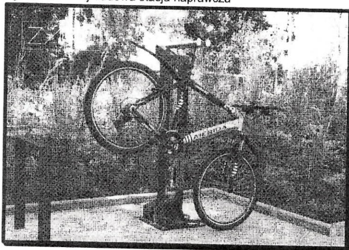
Rysunek 8. Przykładowa stacja naprawcza
